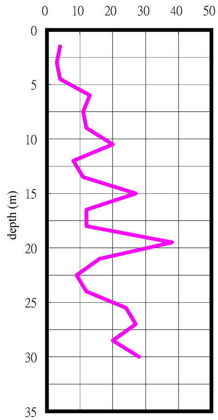
SPT-N
