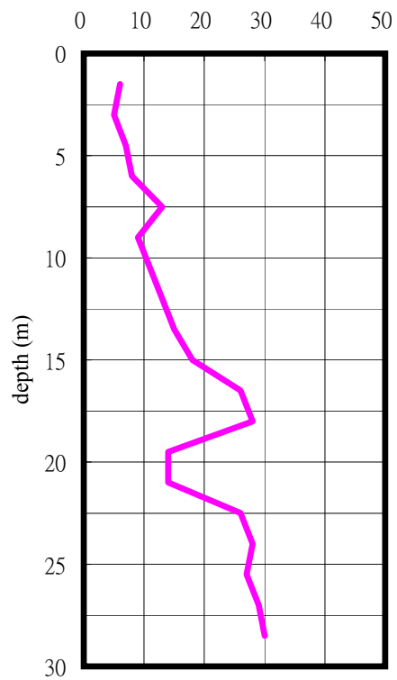
SPT-N
