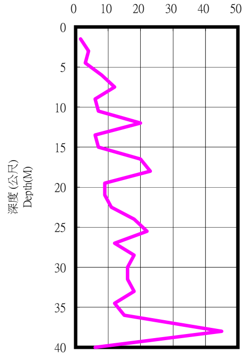
SPT-N
