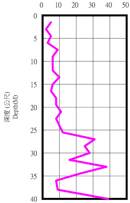
SPT-N
