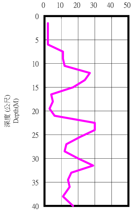
SPT-N
