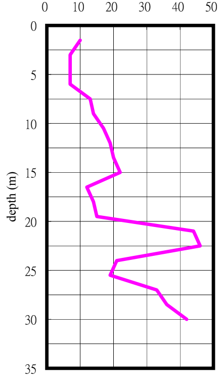
SPT-N
