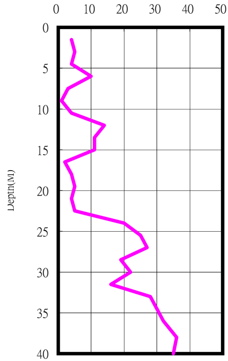
SPT-N
