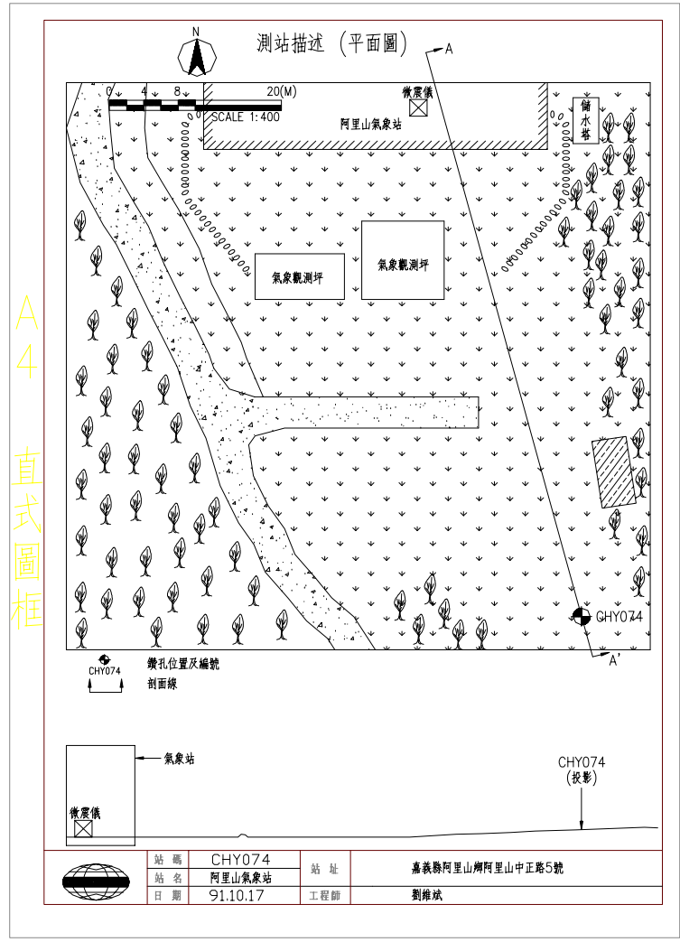
強震儀位置於阿里山氣象站室內，氣象站是日據時代所構築之木造2層樓房，儀器是設置在長×寬×高(3.64×5.45×1.8m)的混凝土基台上。
