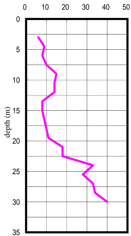
SPT-N
