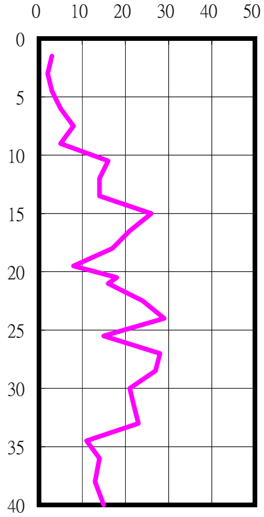
SPT-N
