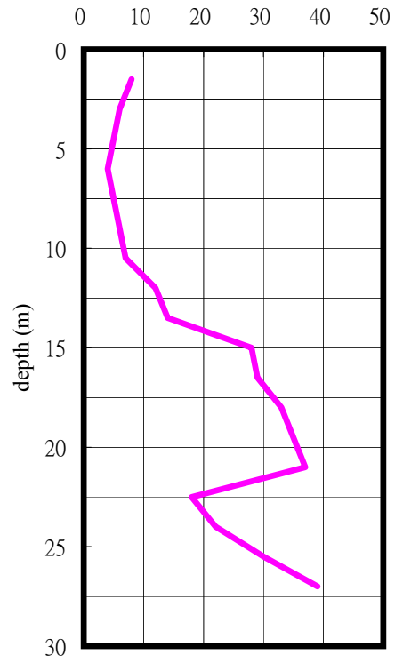
SPT-N
