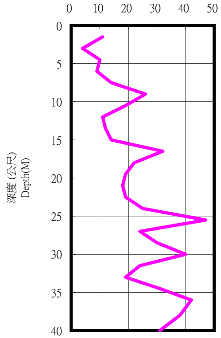
SPT-N
