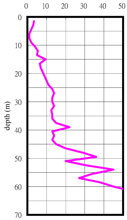
SPT-N
