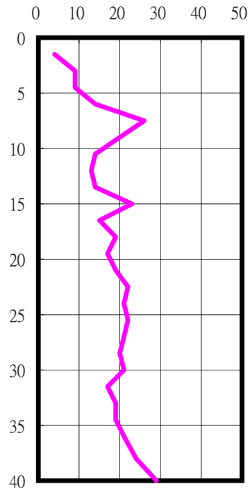
SPT-N
