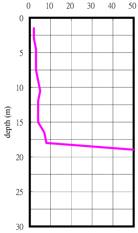
SPT-N
