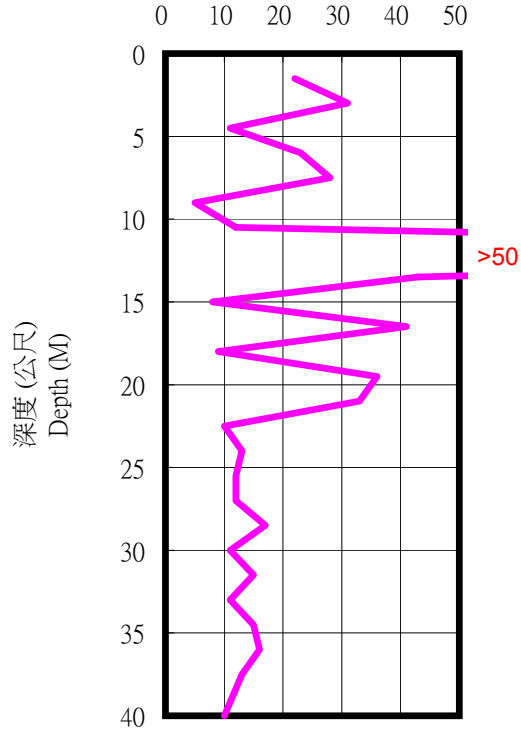
SPT-N
