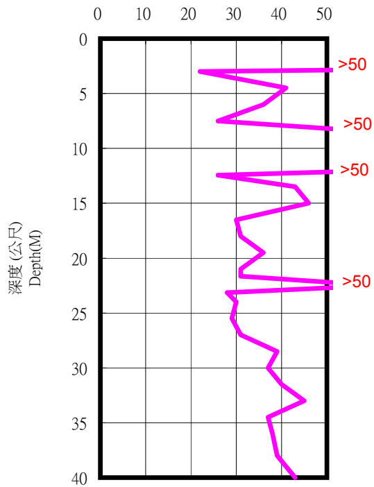
SPT-N
