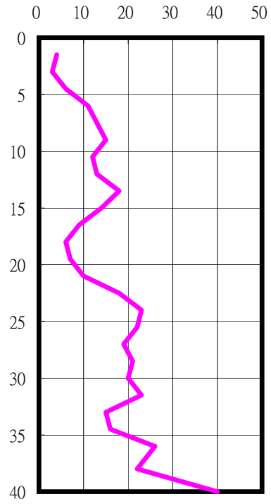
SPT-N
