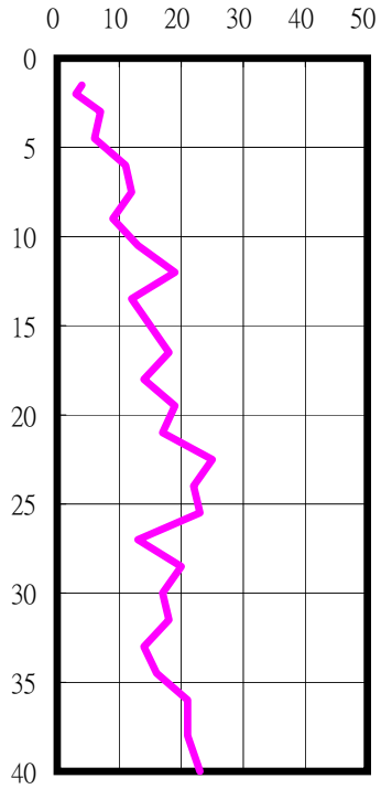
SPT-N
