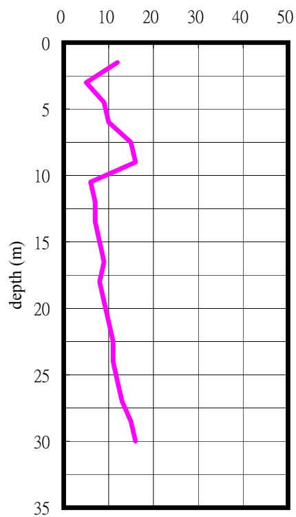
SPT-N
