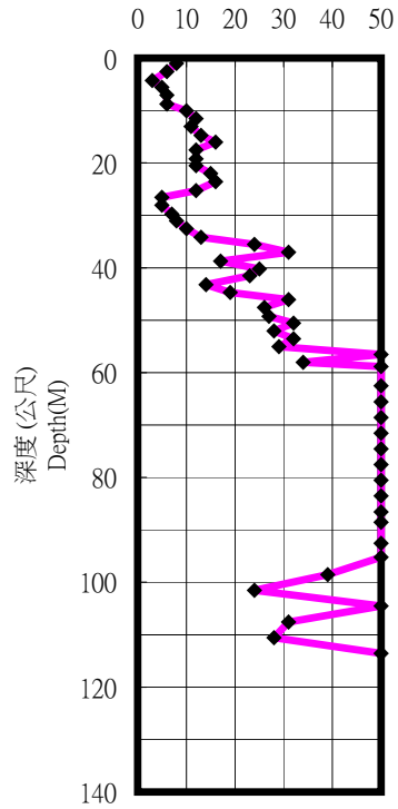
SPT-N
