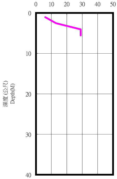
SPT-N
