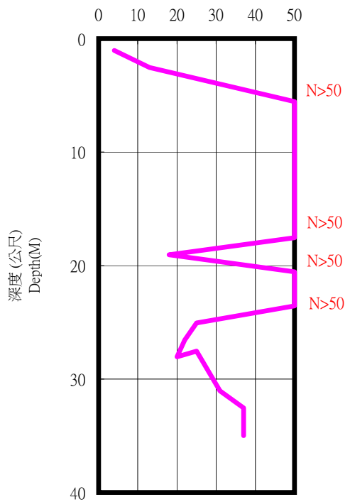
SPT-N
